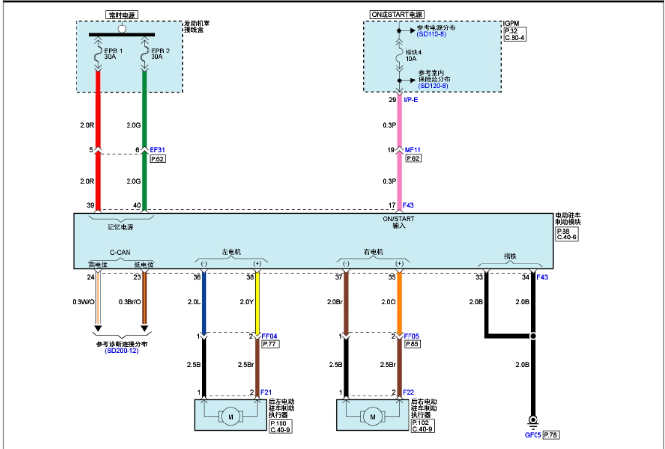
电动驻车制动(EPB)系统(2)
